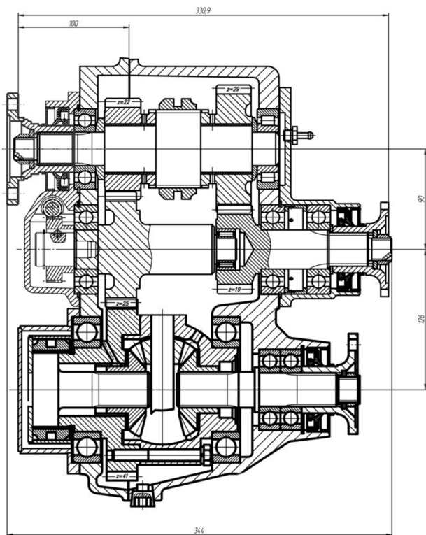
Рис. 6.11 Коробка привода заднего ведущего моста с приводом водометного двигателя
