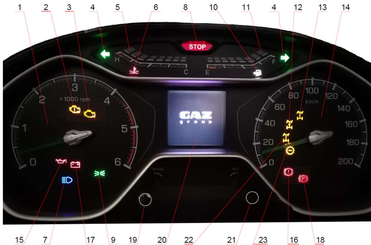
Рис. 5.4 Комбинация приборов (вариант 2)
